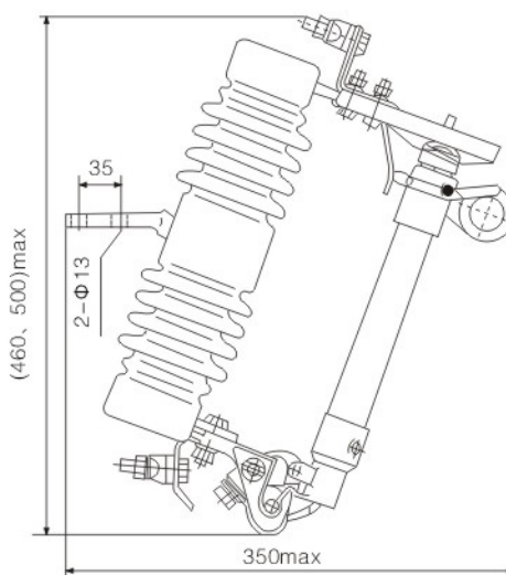
PRW8-12(III, IV)/200型熔断器 PRW8-12(II,IV)/200 dropout fuse
